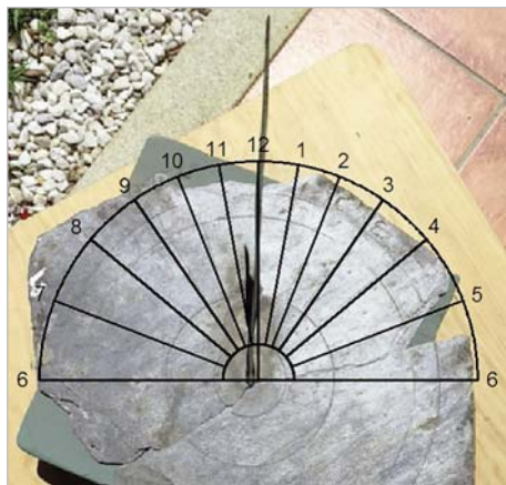
Cálculo de horas do reloxo horizontal
