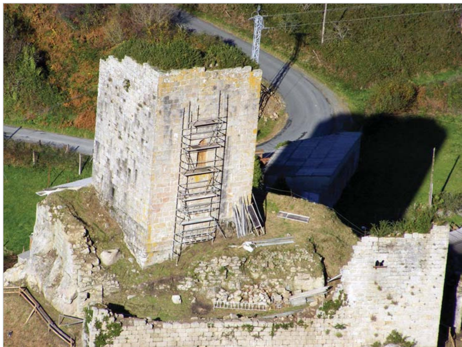
Fig. 54. Perspectiva sur da torre da homenaxe previa á intervención da 2ª fase
