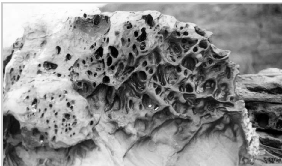
Filigranas sobre o xisto que a erosión fai na cara interior da canle da illa de Máis á Terra, no arquipélago do Carbón.
