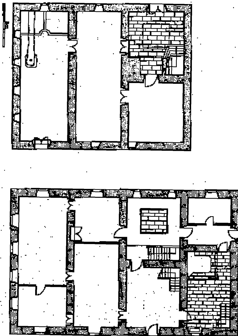
Fig. 10. Plantas baja y principal del pazo. (Pazos de Galicia, vol. I, 24).
