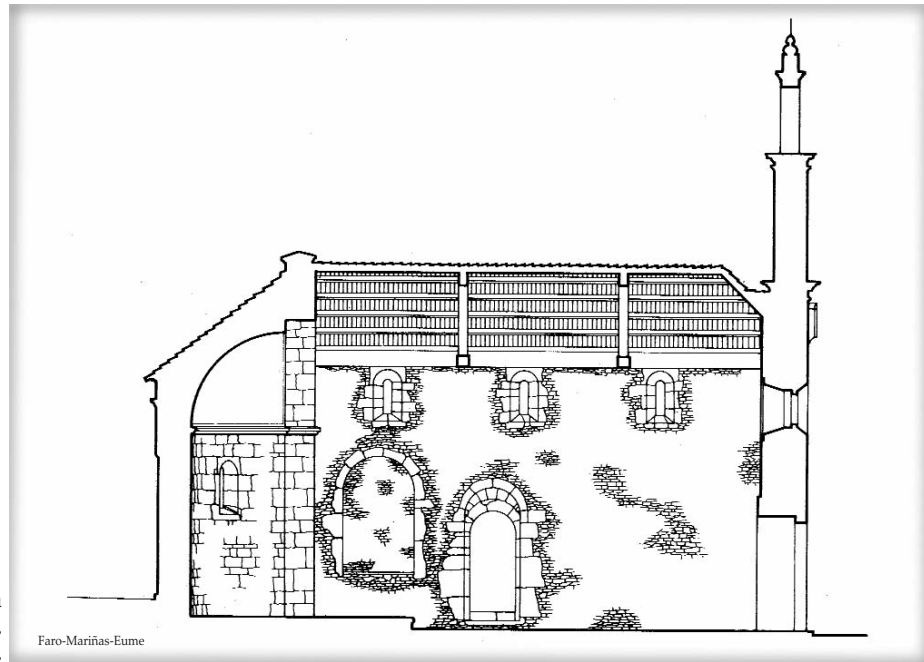
San Xoán de Vilanova. Sección lonxitudinal.
