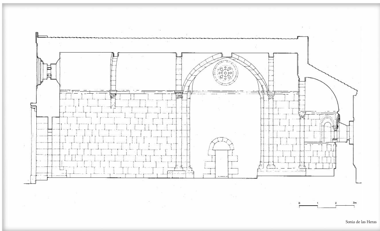
Sección lonxitudinal de San Miguel de Breamo
