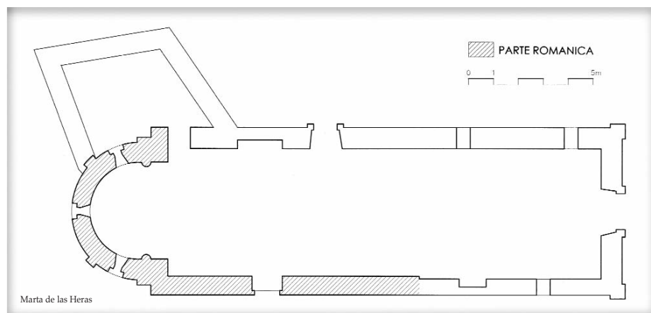
Planta de San Martíño de Andrade.
